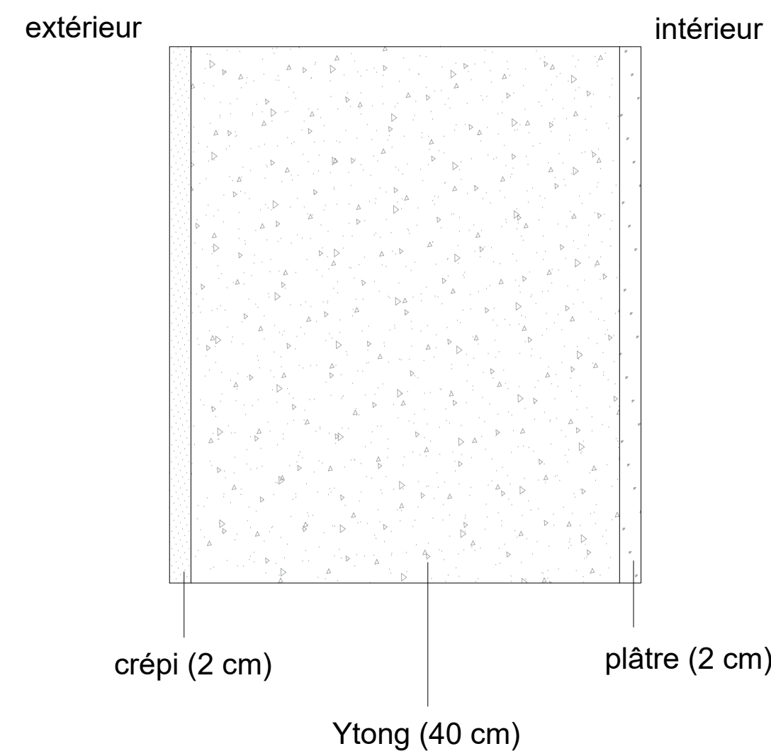
schéma mur extérieur
