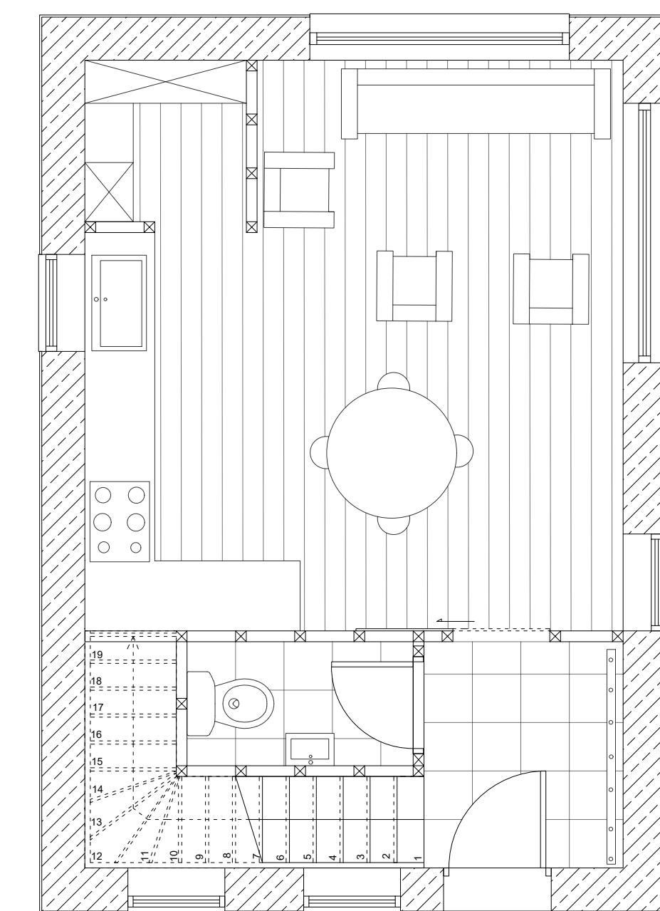
PLAN R0 1 / 50
