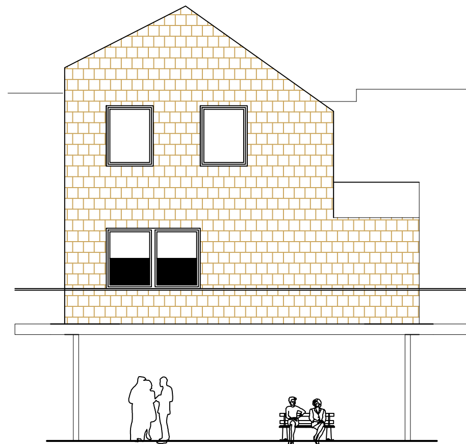
Elevation est 1/100
