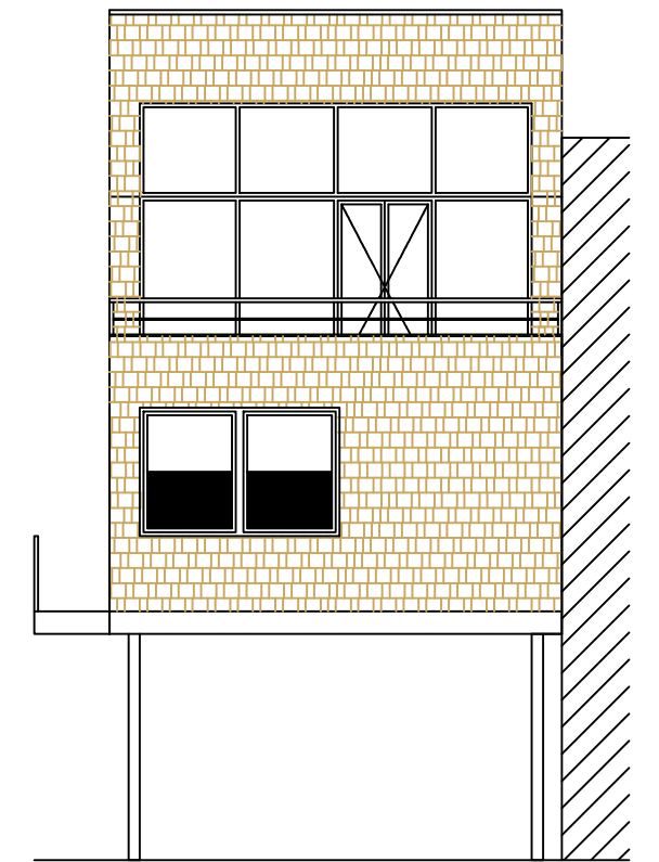
Elevation Sud 1/100
