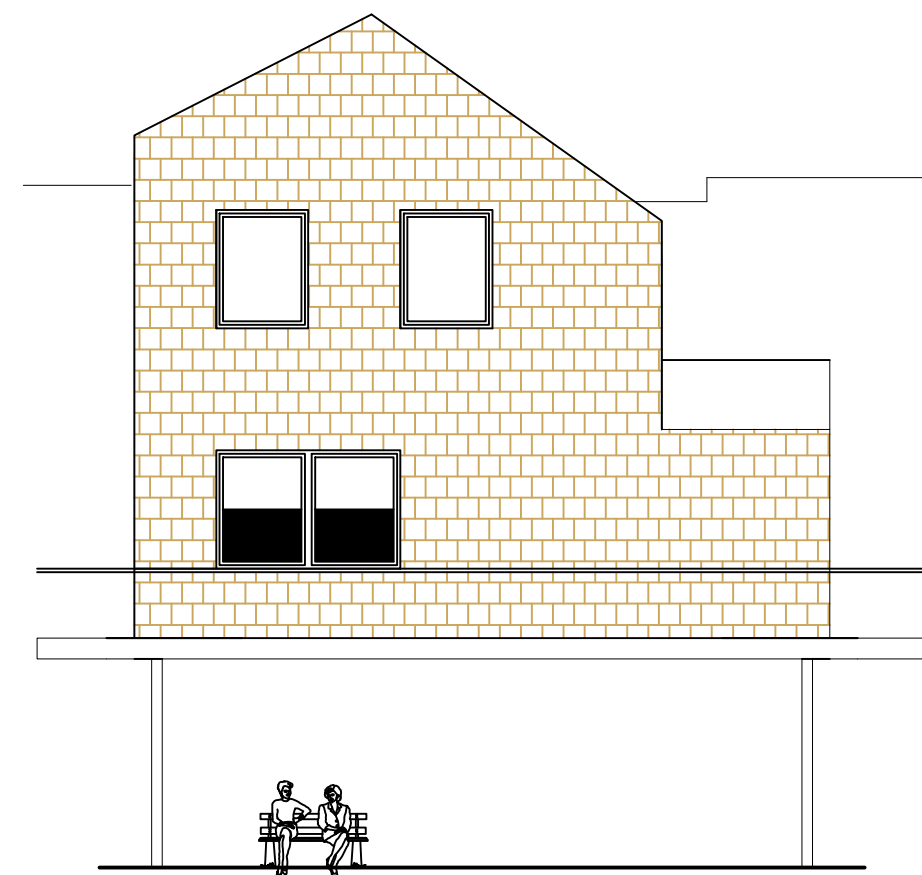
Elevation est 1/100
