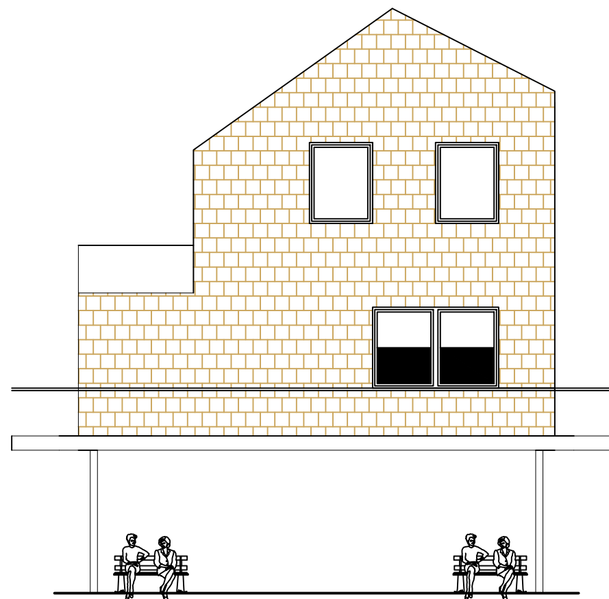
Elevation ouest 1/100
