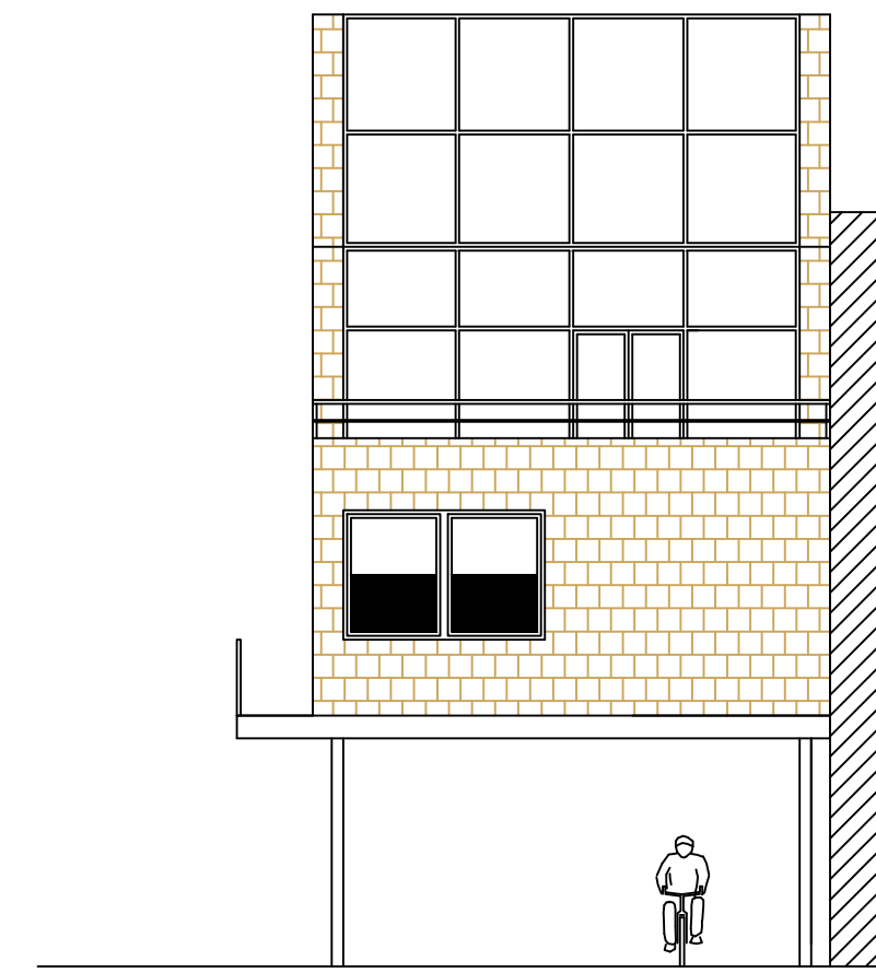
Elevation Sud 1/100
