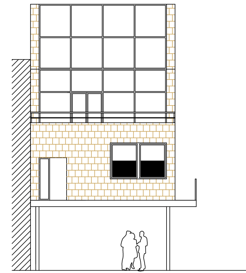
Elevation Sud 1/100
