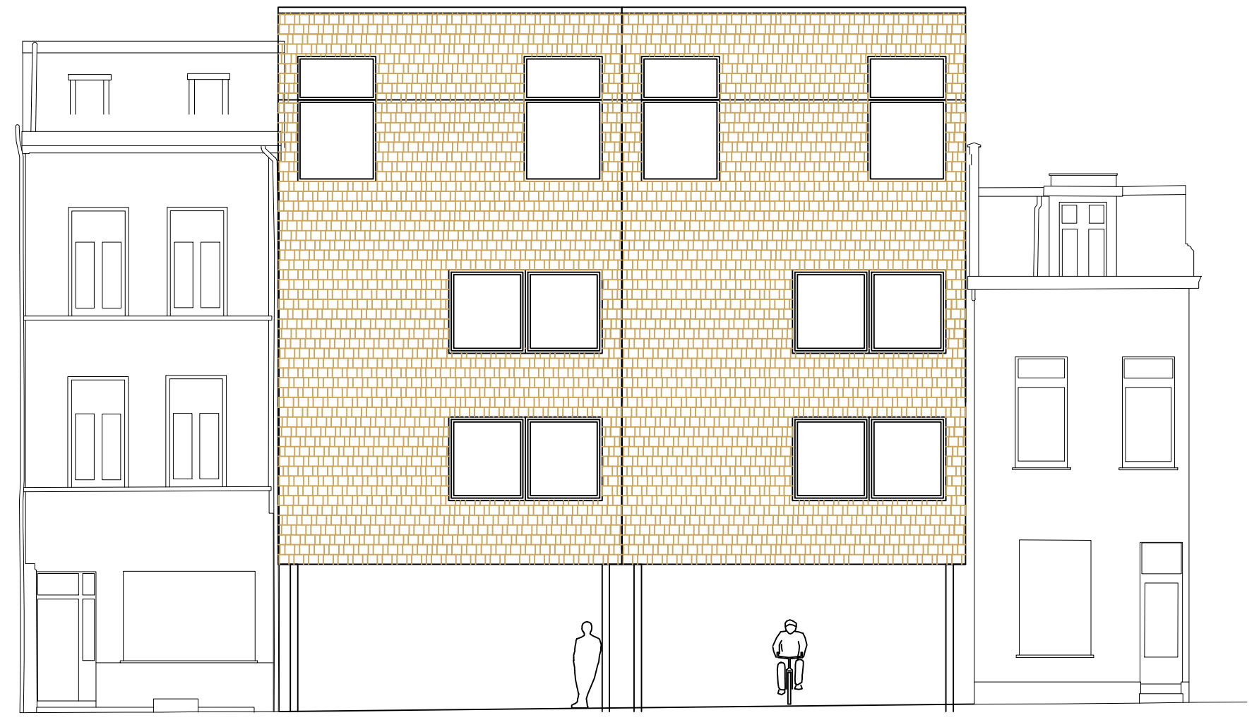
Elevation Nord 1/100
