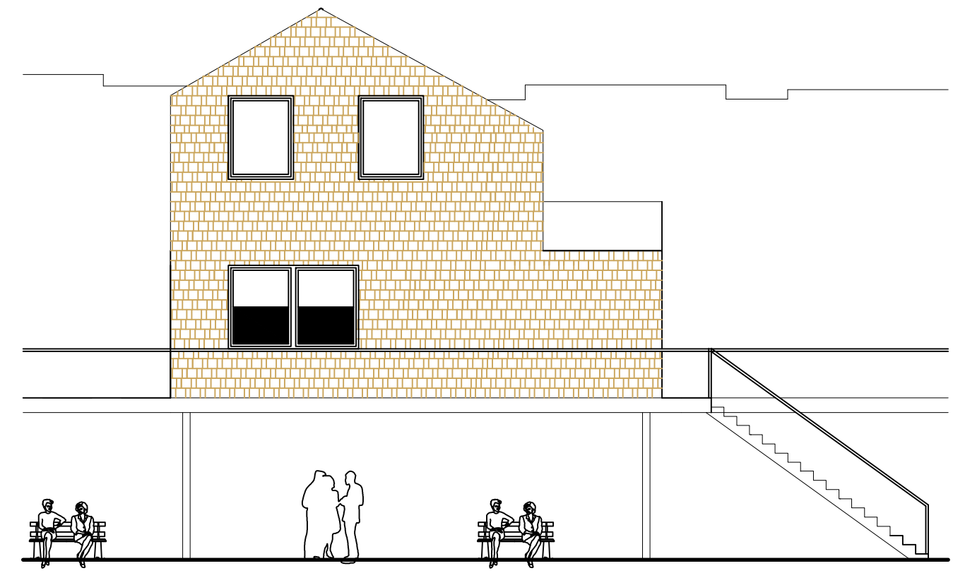
Elevation est 1/100
